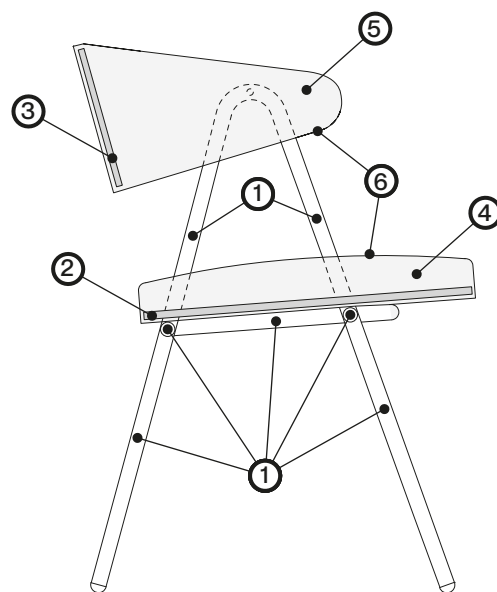
SEZIONE A-A
